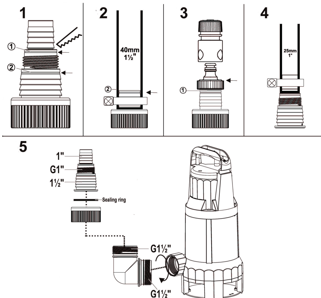
Abb. 5-3: Schlauchanschluss
